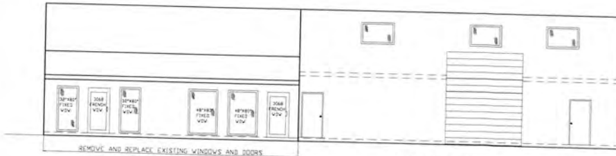
FRONT ELEVATION SCALE: 1/8" = 1'-0"
