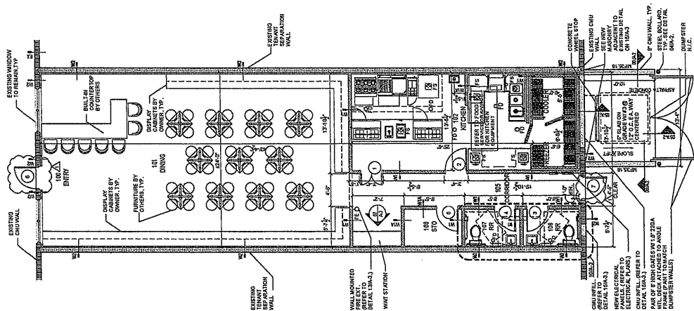
01 FLOOR PLAN SCALE: 1/8" = 1'-0"
