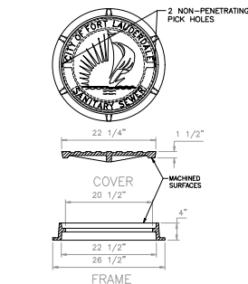
200 MANHOLE FRAME & COVER PAVED AREAS N.T.S.
