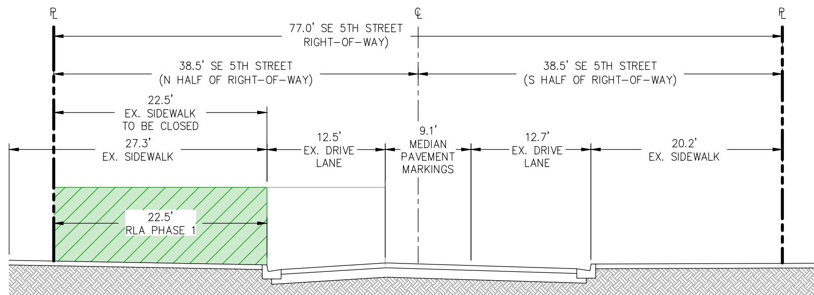
SECTION B-B RLA PHASE 1 N.T.S.
