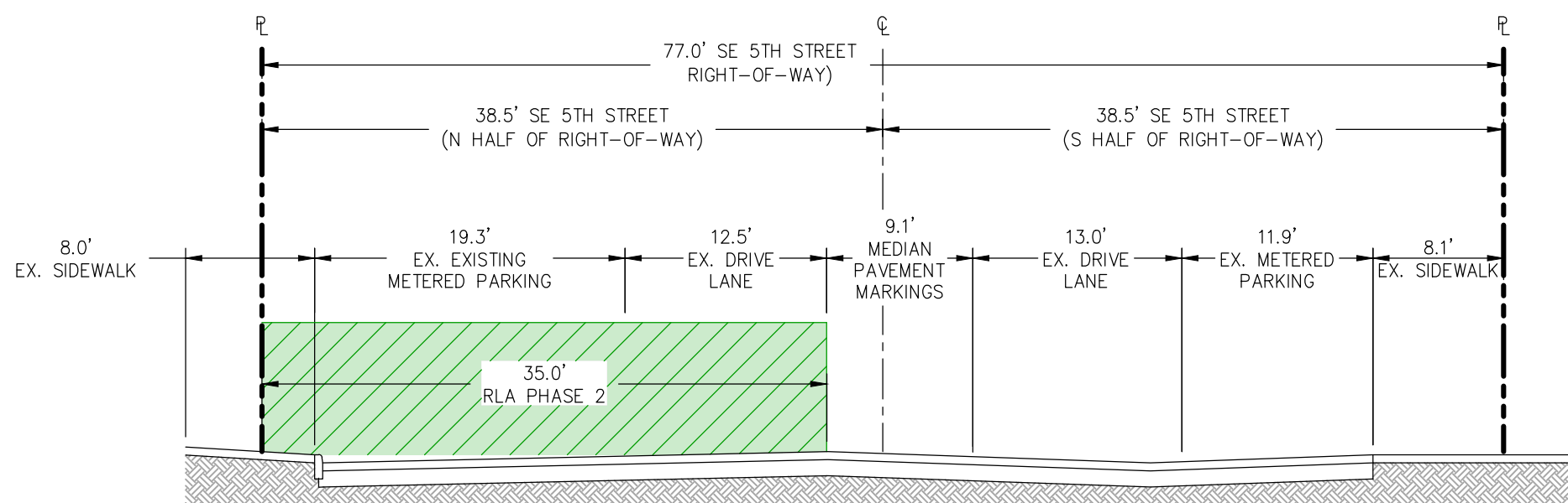
SECTION A-A RLA PHASE 2 N.T.S.
