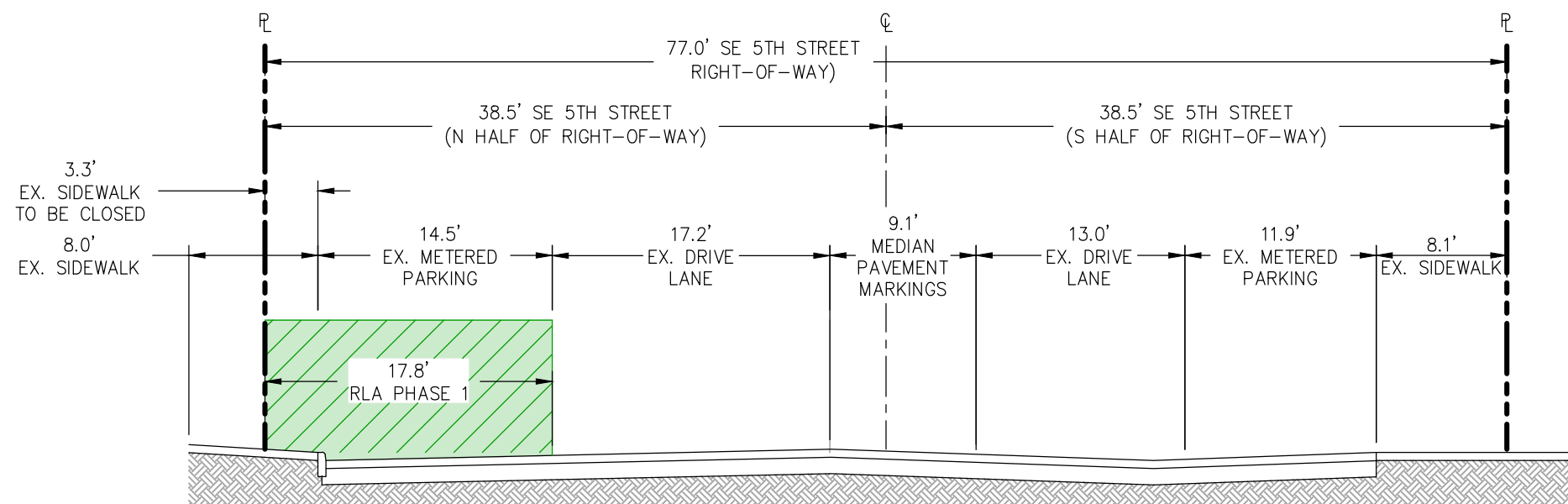
SECTION A-A RLA PHASE 1 N.T.S.
