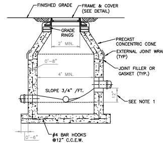
204 SHALLOW MANHOLE N.T.S.
