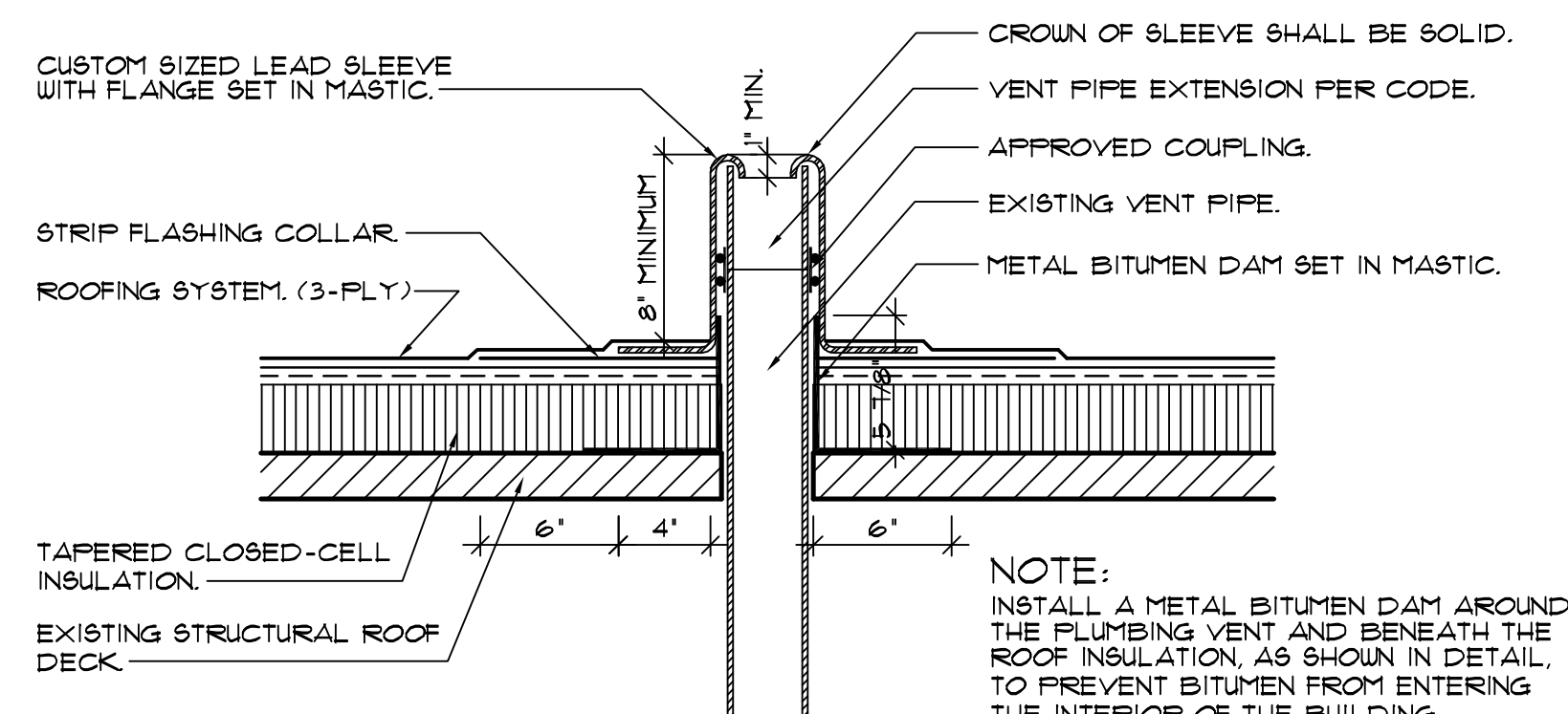
2 A-3 PLUMBING VENT DETAIL SCALE: 1/2" = 1'-0"
