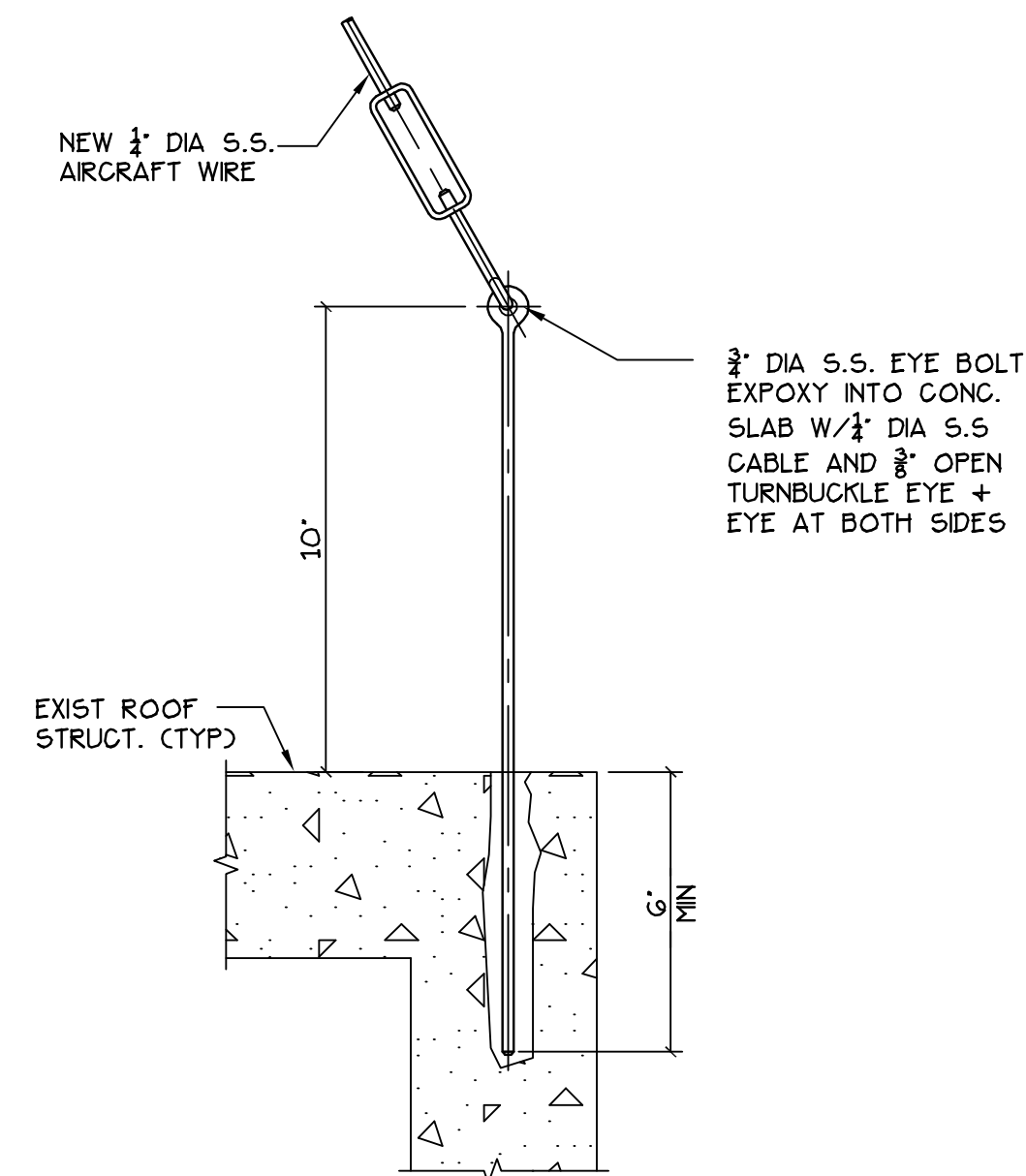
ANCHOR DETAIL SCALE: 3"=1'-0"
