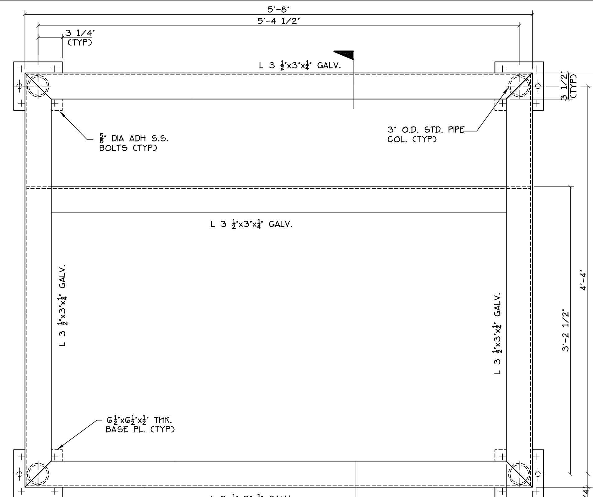
ANCHOR DETAIL SCALE: 3"=1'-0"
